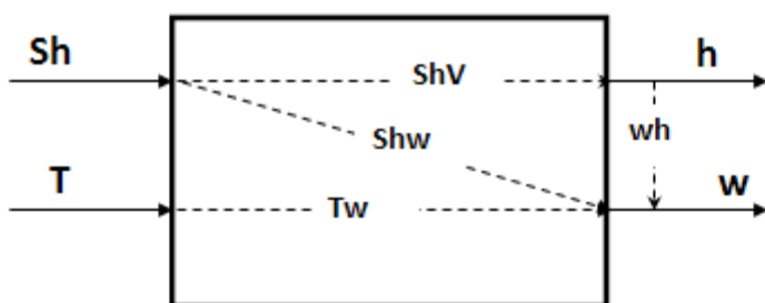
Схема 2. Сигнали вхід-вихід зерносушарки каскадного типу з киплячим шаром
