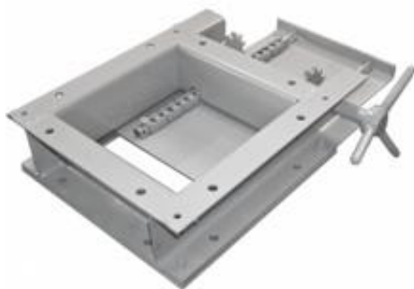
Заслінка шиберу
