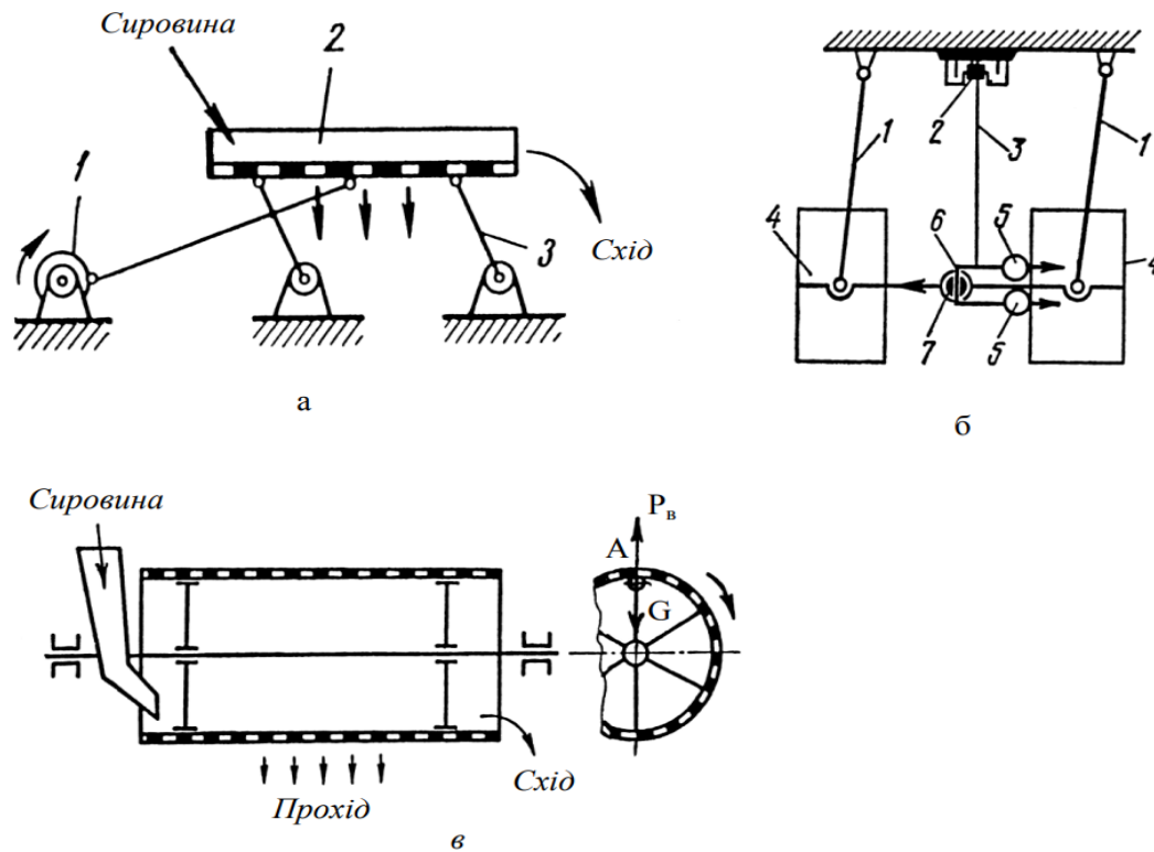
Рис. 1. Схеми машин для просіювання (сита): а - з поступальним рухом; б - з коловим поступальним рухом; в — з обертальним рухом.
