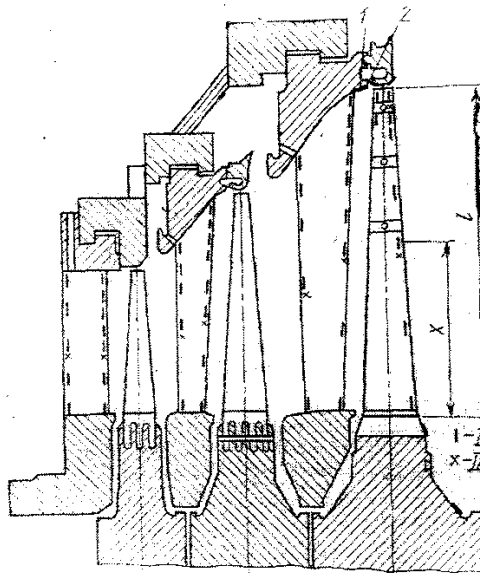
Рисунок 2. Розташування датчиків.
