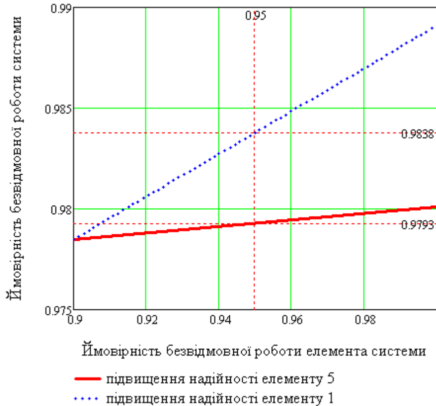
Рисунок 3. Залежність ймовірності безвідмовної роботи системи від ймовірності безвідмовної роботи її складових при використанні методу гіпотез
