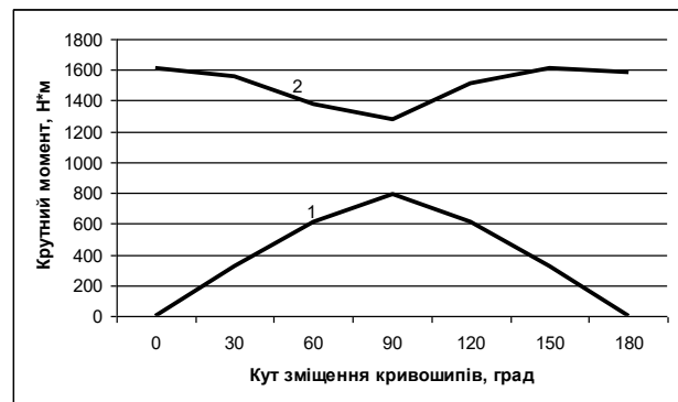
Рисунок 3. Графіки зміни мінімального (1) та максимального (2) значень зведеного моменту статичного опору в залежності від кута зміщення кривошипів
