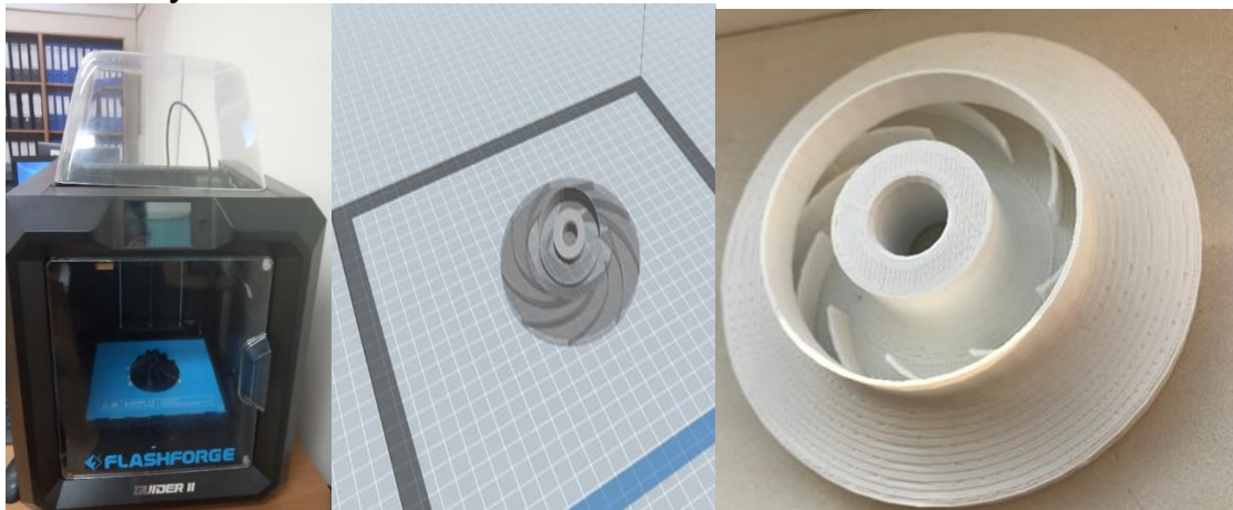
Рисунок 8 3D-принтер для изготовления прототипов моделей центробежных колес
