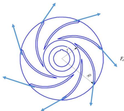
Рисунок 5 Вычислительная схема для статического анализа напряженно-деформированного состояния колеса (SSS)
