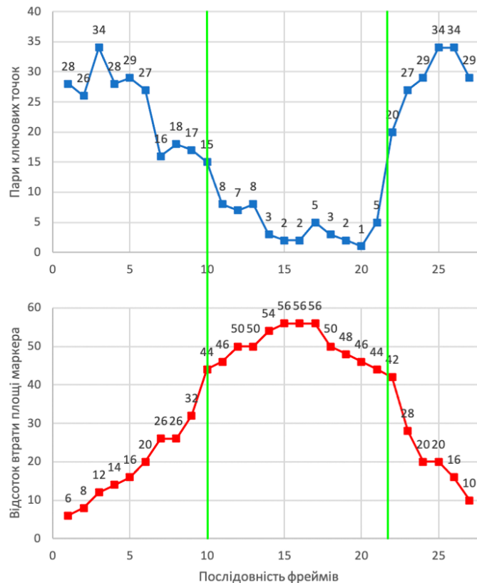
Рис. 3. Залежність наявної частини маркера, що присутня на оригінальному зображенні, від кількості знайдений пар ключових точок.
