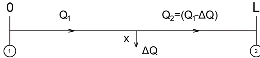
Рис. 1. Принципова гідравлічна схема для моделювання односточкового витоку на ділянці напірного трубопроводу
