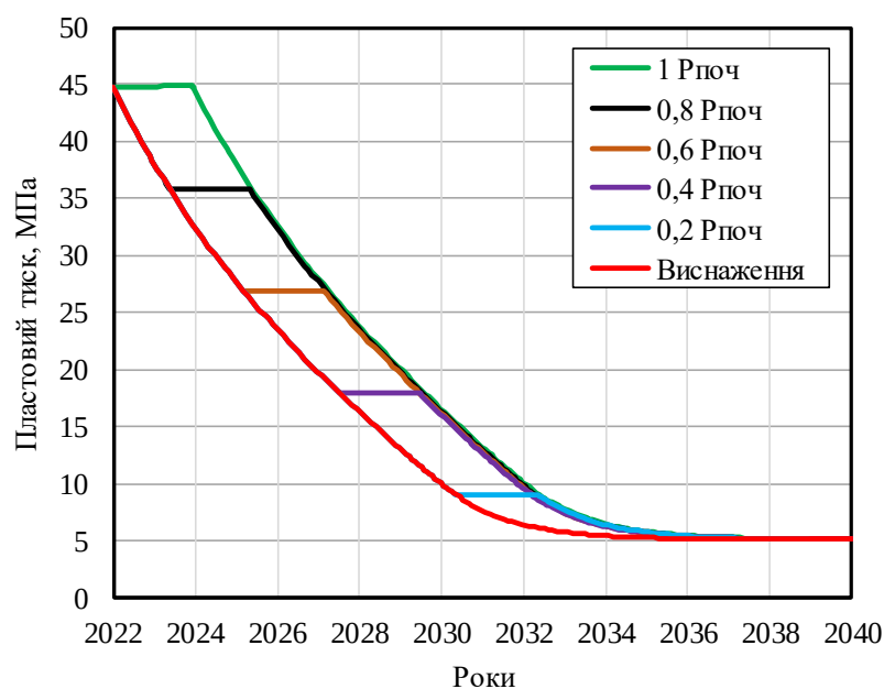
Рисунок 1 –Динаміка пластового тиску від тиску початку нагнітання сухого газу в газоконденсатний поклад та при розробці на виснаження
