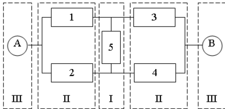
Рисунок 1. Логічна схема розрахунку надійності телекомунікаційної мережі
