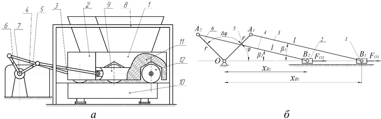
Рисунок 1. Роликова формувальна установка з рекупераційним приводом (а) та її кінематична схема (б).
