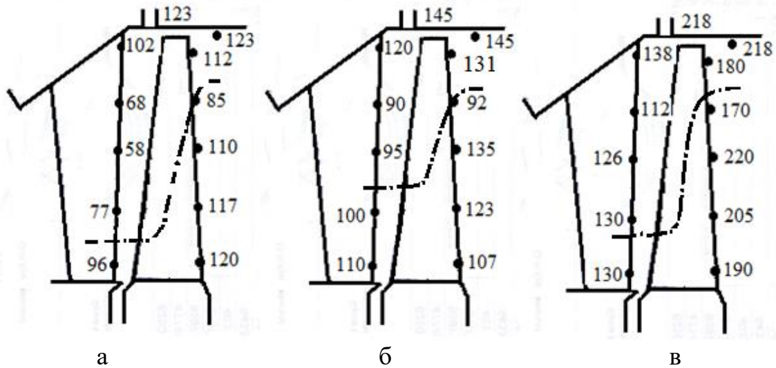
Рисунок 3. Розподіл температури пари у 31-му ступені турбіни Т-250/300-240: а – P_k = 9,8 кПа, G = 23,9 кг/с; б – P_k = 19,6 кПа, G = 24,7 кг/с; в – P_k = 24,9 кПа, G = 20,8 кг/с.
