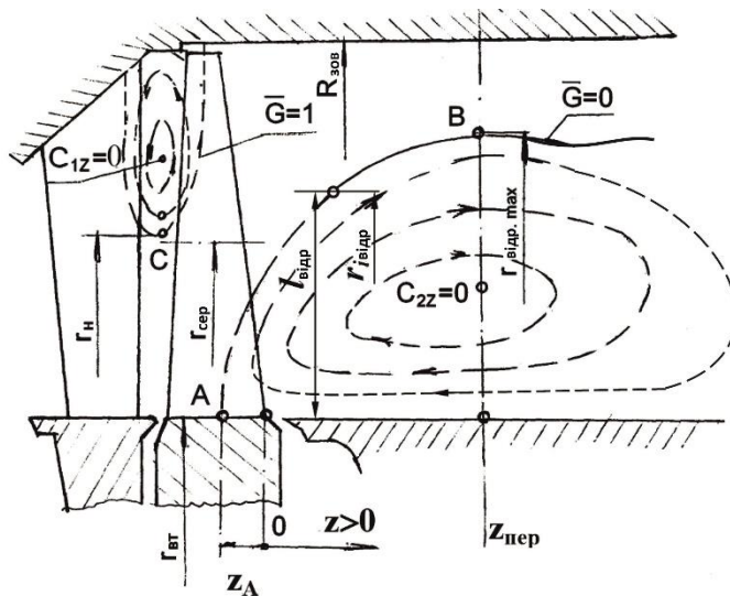
Рисунок 1. Основні геометричні характеристики області привтулкового відриву і вихору, що обертається у ступені.
