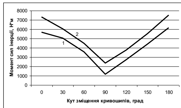
Рисунок 5. Графіки зміни відхилень зведеного моменту від сил інерції \Delta M_{i\max} (1) та \Delta M_i (2) в залежності від кута зміщення кривошипів
