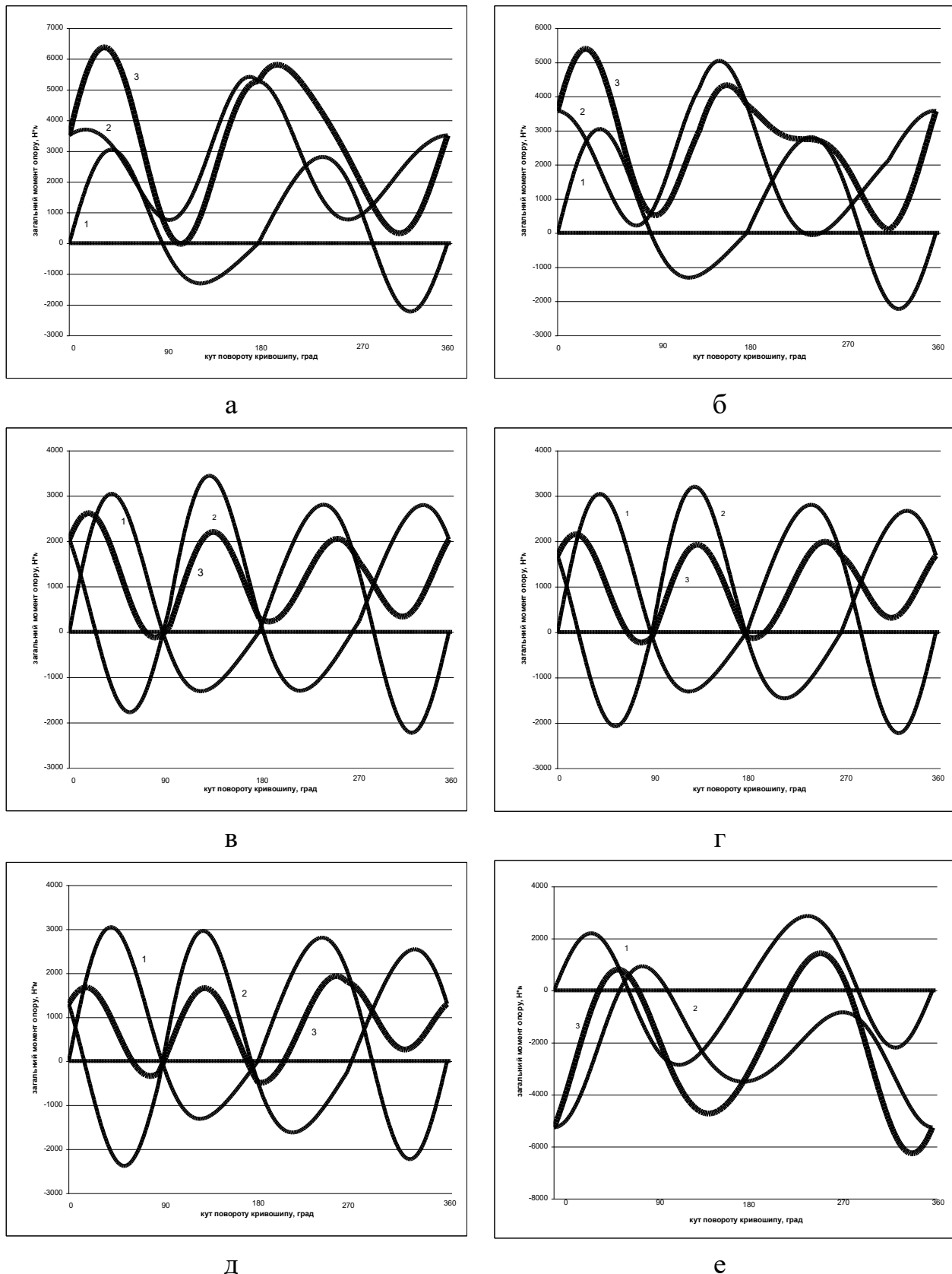
Рисунок 6. Графіки зміни загального моменту сил опору на привідному валу установки при різних значеннях кута зміщення кривошипів: а – \Delta\varphi = 0^\circ ; б – \Delta\varphi = 45^\circ ; в – \Delta\varphi = 85^\circ ; г – \Delta\varphi = 90^\circ ; д – \Delta\varphi = 95^\circ ; е – \Delta\varphi = 180^\circ ; 1, 2 – загальні моменти сил опору першого та другого візків відповідно; 3 – сумарний момент сил опору
