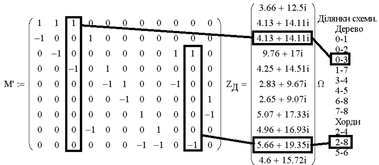
Рисунок 2. Урахування конфігурації схеми мережі
