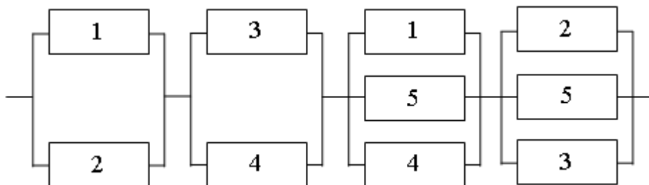
Рисунок 5. Логічна схема надійності за методом перетинів
