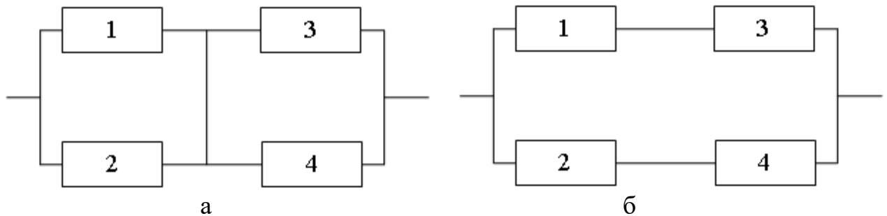
Рисунок 2. Логічна схема розрахунку надійності за методом гіпотез: а – абсолютно надійний елемент 5; б – абсолютно ненадійний елемент 5
