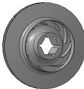
Рисунок 2 3D-модель рабочего колеса центробежного насоса (СР) с цилиндрическими лопатками
