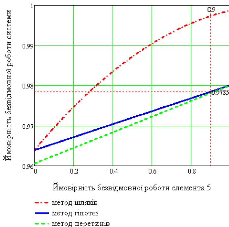
Рисунок 6. Залежність ймовірності безвідмовної роботи системи від ймовірності безвідмовної роботи мостового елемента при використанні методу гіпотез, шляхів та перетинів
