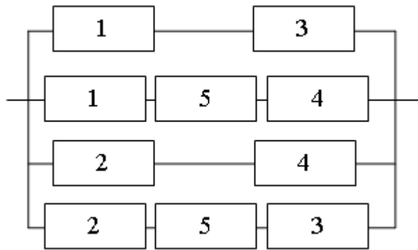
Рисунок 4. Логічна схема надійності за методом шляхів
