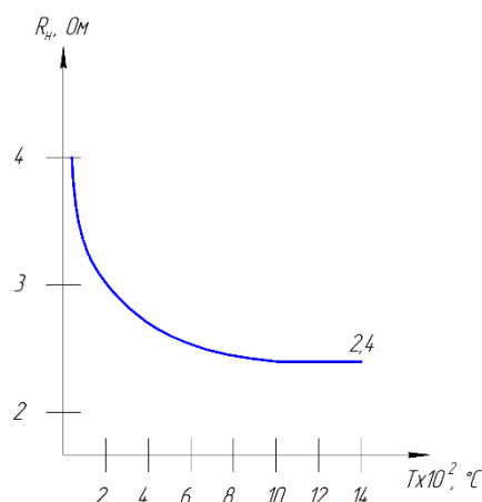
Рисунок 2. Графік залежності опору резистивного нагрівача від температури
