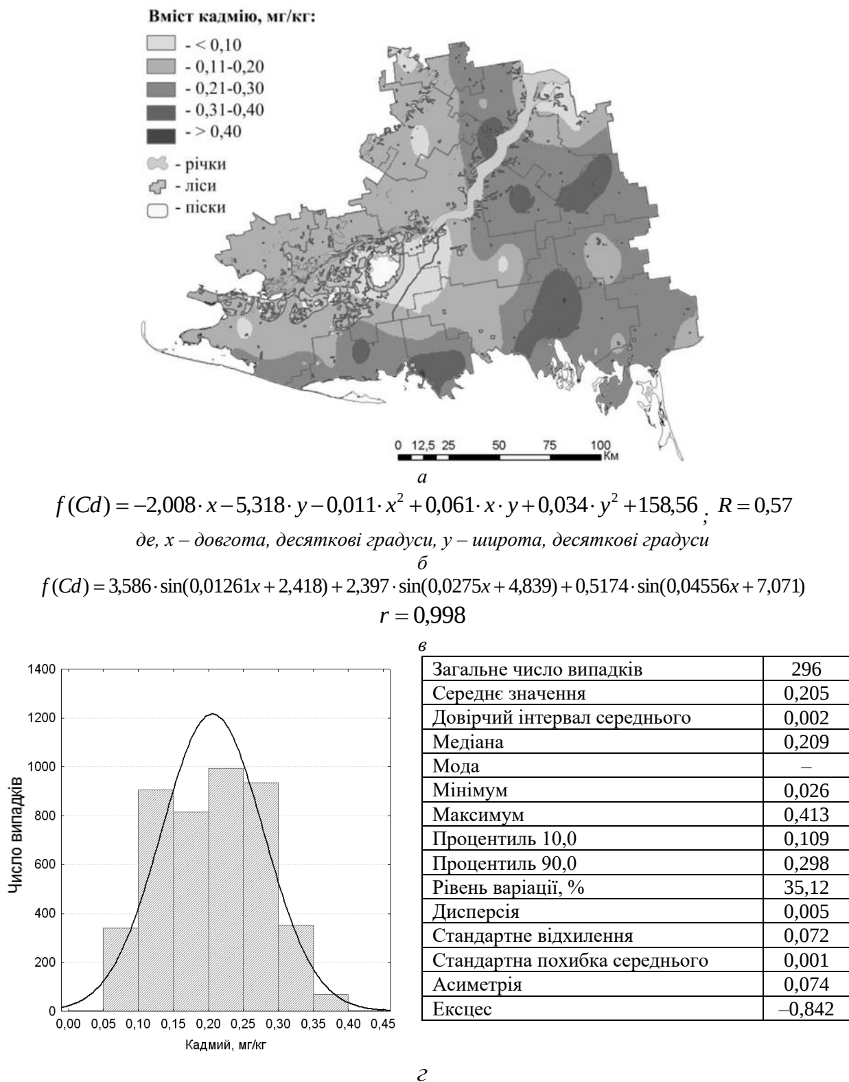
Рисунок 13. Статистично–картографічні характеристики розподілу кадмію в шарі 0...20 см ґрунту Херсонської області: а – картограма розподілу;
